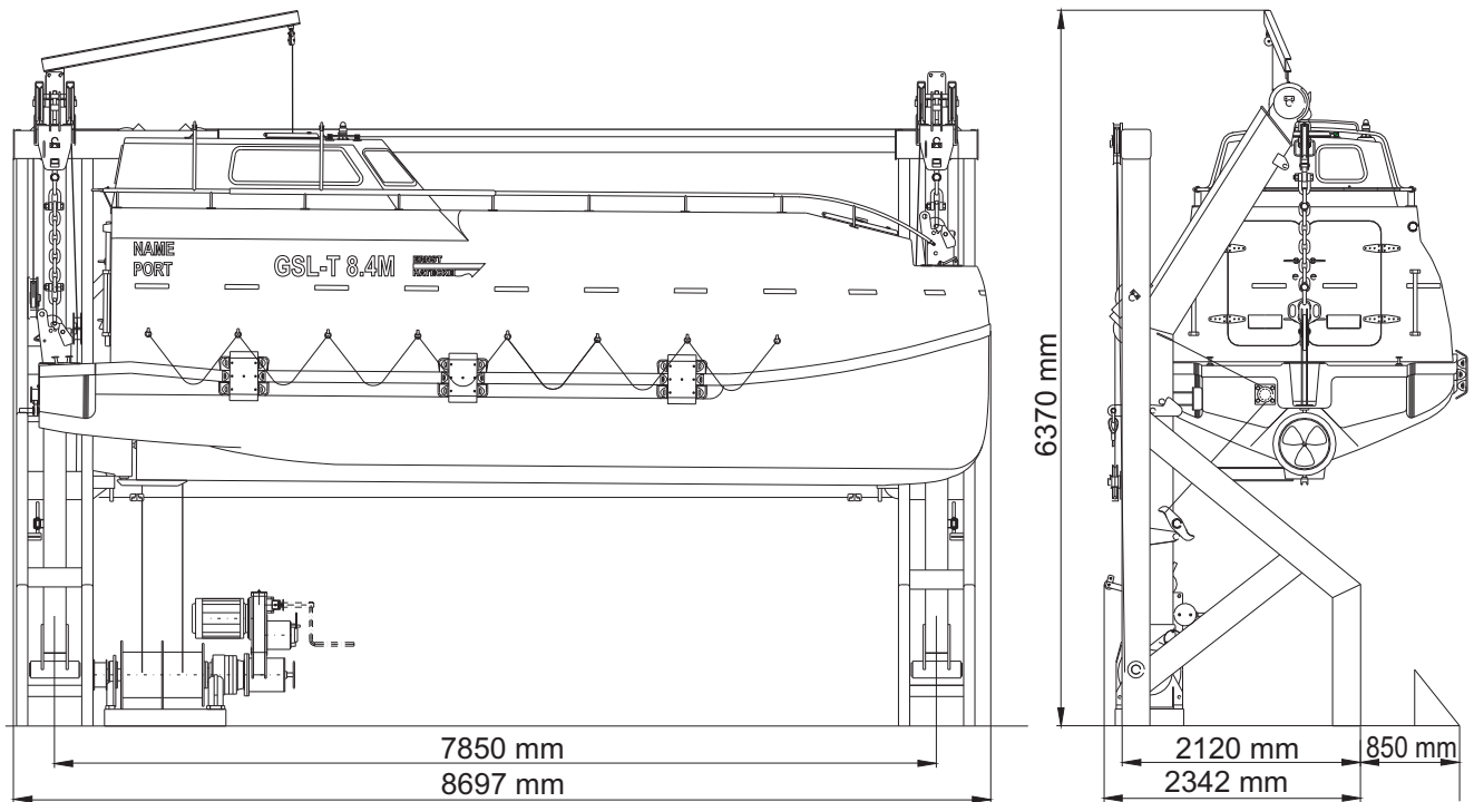
scale 1 : 75
